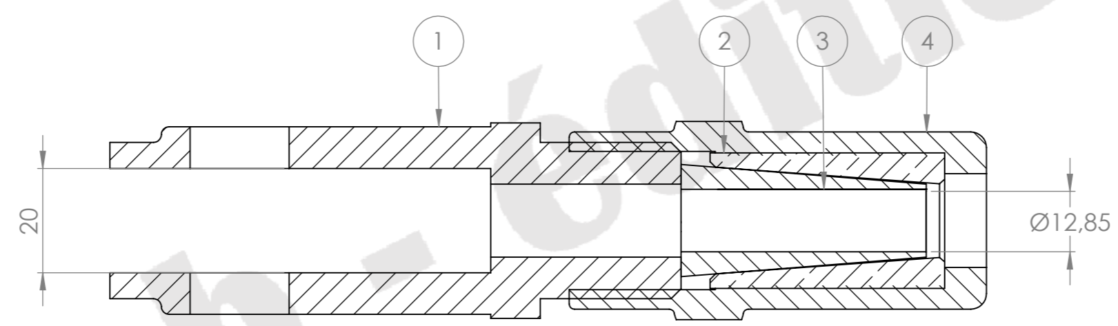
COUPE A-A ECHELLE 1 : 1
