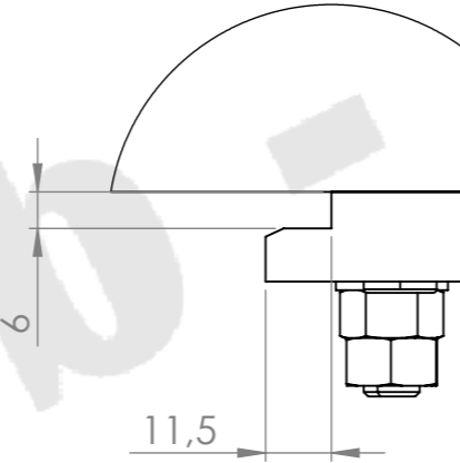
DÉTAIL A ECHELLE 1 : 1.5
